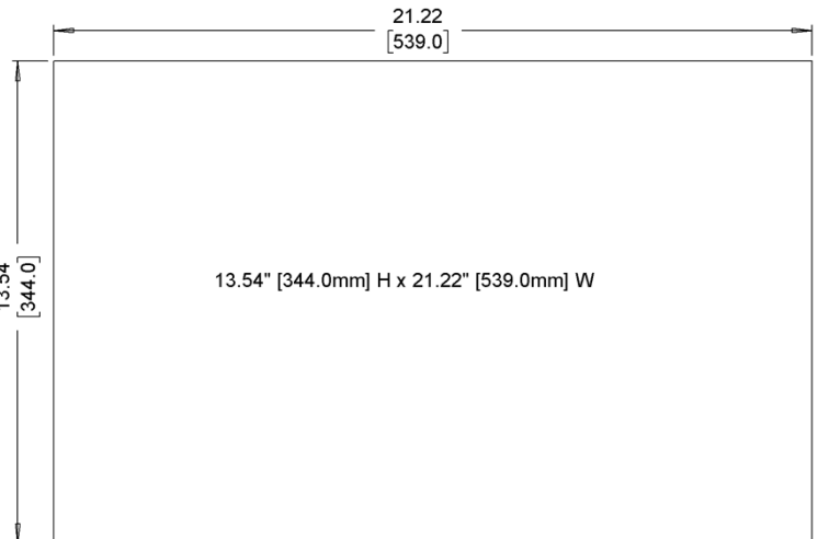
Cutout Dimensions
