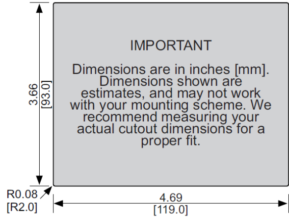
Cutout Dimensions
