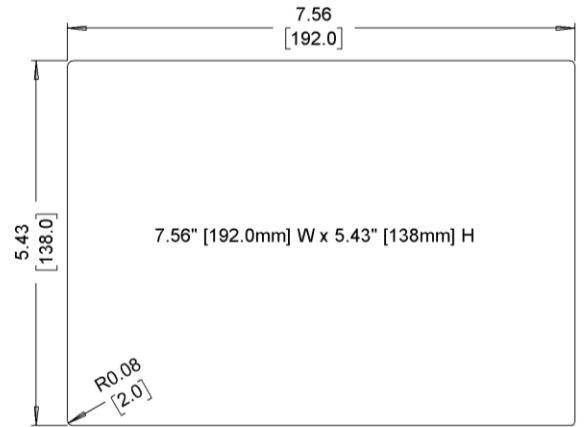
Cutout Dimensions
