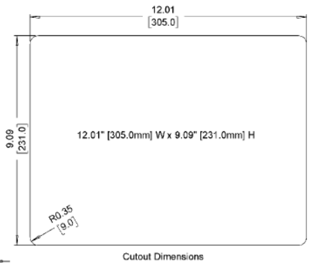
Cutout Dimensions
