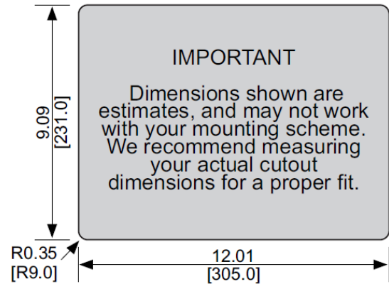
Cutout Dimensions
