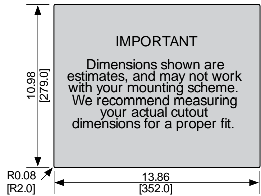
Cutout Dimensions
