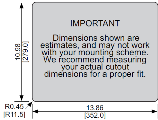
Cutout Dimensions
