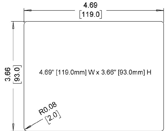
Cutout Dimensions
