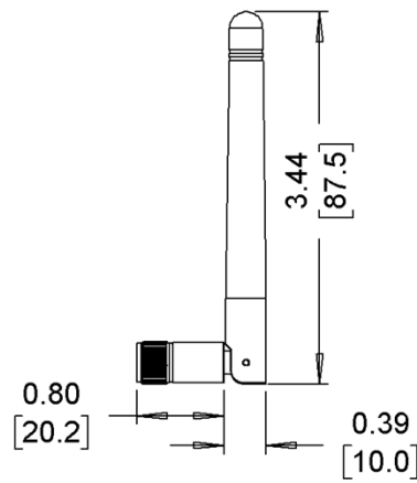
Antenna
