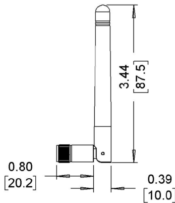
Antenna
