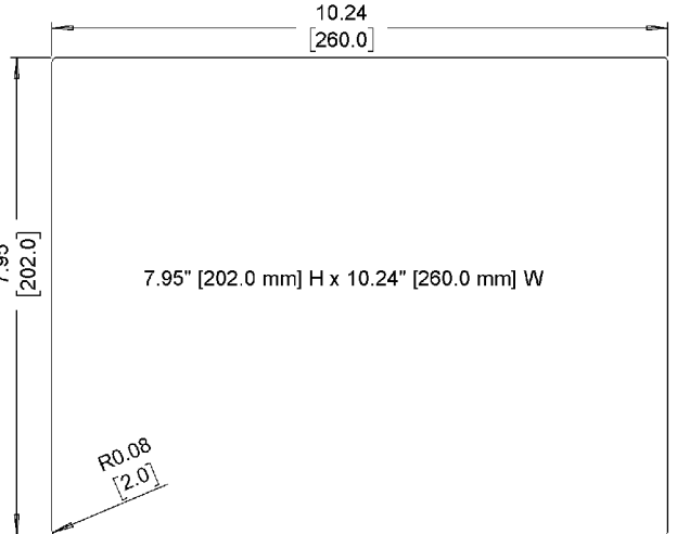
Cutout Dimensions
