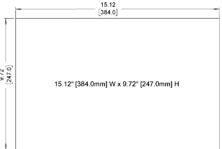
Cutout Dimensions
