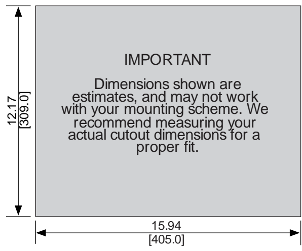
Cutout Dimensions
