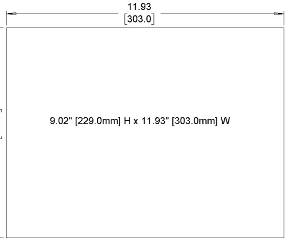
Cutout Dimensions
