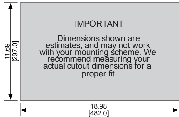
Cutout Dimensions
